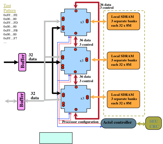
Fig. 2. RCC Module Diagram
